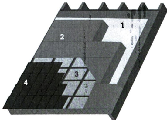
1. Dampscherm | 2. Isolatie | 3. Onderdak | 4. Dakbekleding
