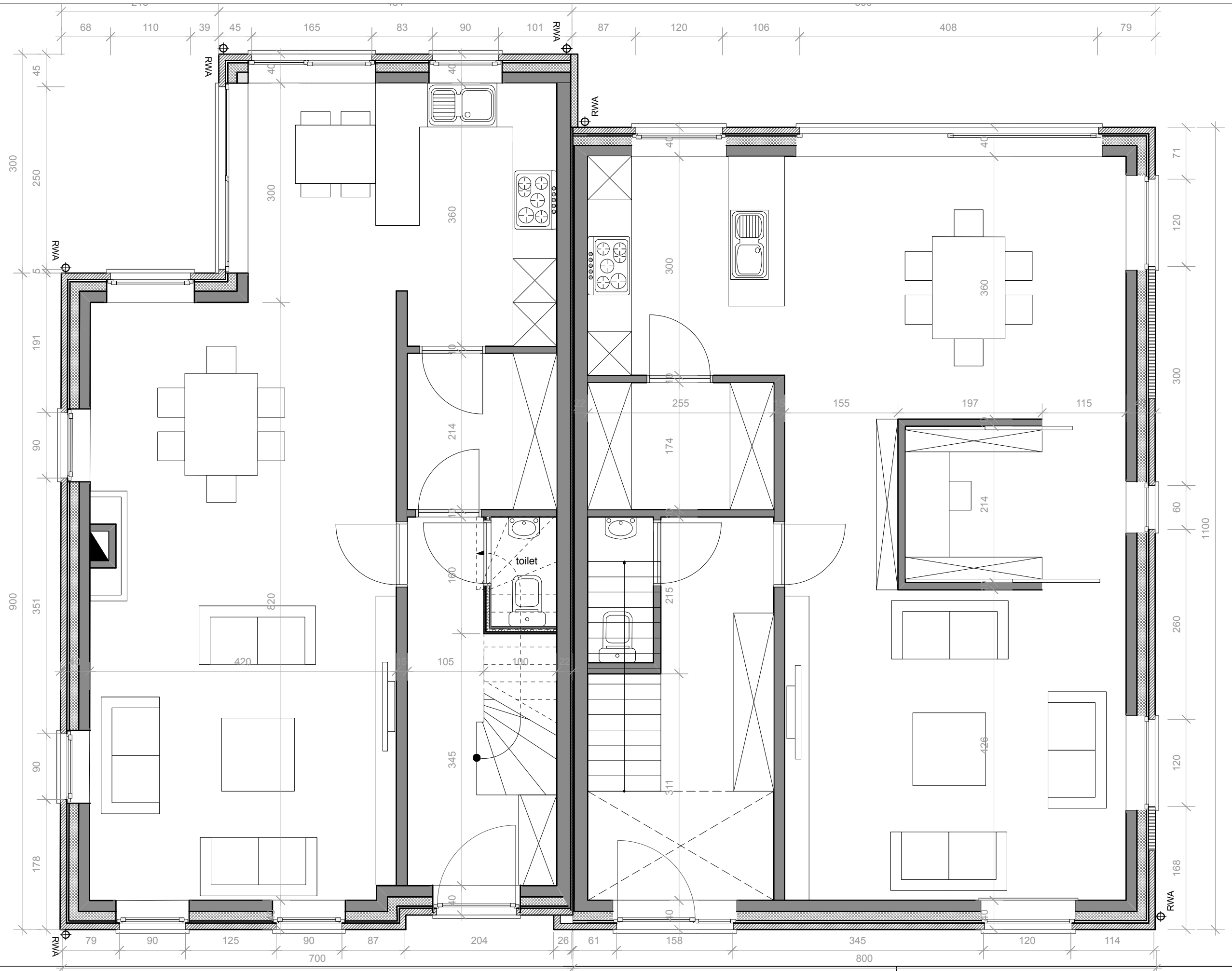
PLAN GELIJKVLOERSE VERDIEPING HOB schaal 1/50
